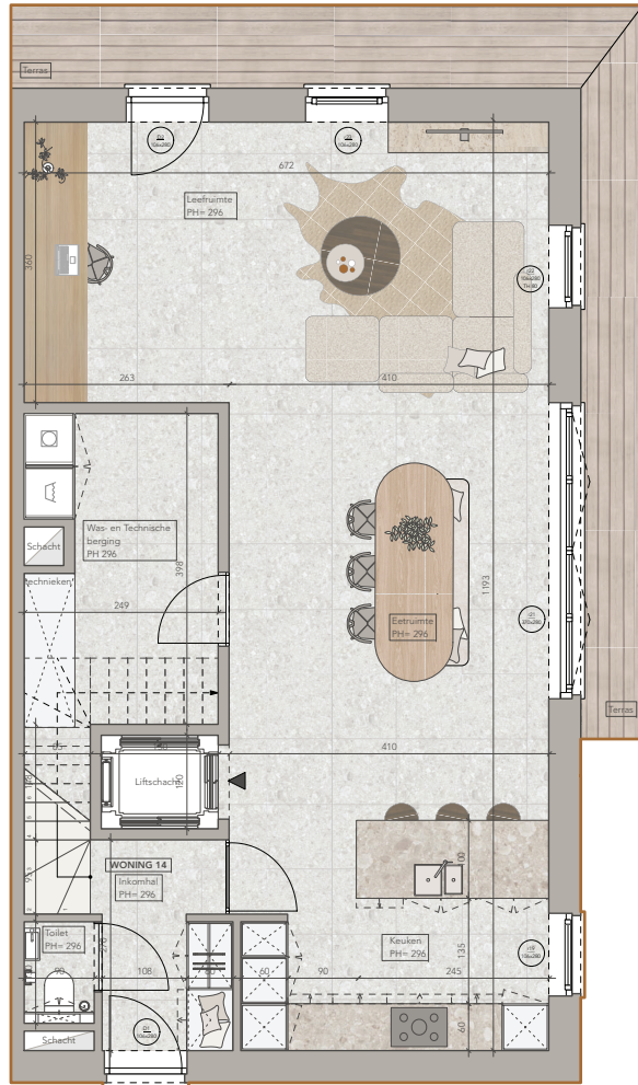
Grondplan LOFTWONING 14
